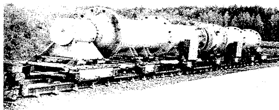
2. ábra • Hengeralakú detonációs nanogyémánt-előállító reaktor (VNTIIF, Sznyezsinszk, Szibéria, Szovjetunió), átmérő: 1,5; hossz: 12 m, töltet: 40 kg (Picardi, 2008).
