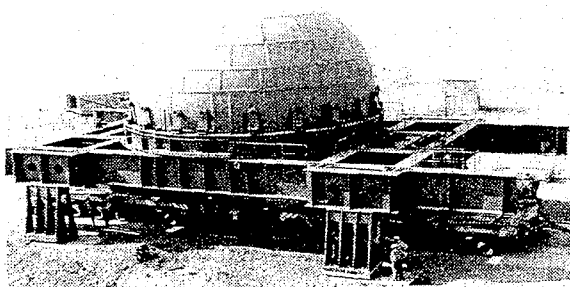
3. ábra • Kupolaalakú detonációs nanogyémántokat gyártó reaktor (VNIIF, Szarov, Szovjetunió), átmérő: 12 m, súly: 350 tonna, töltet: 1 tonna. (Picardi, 2008).
